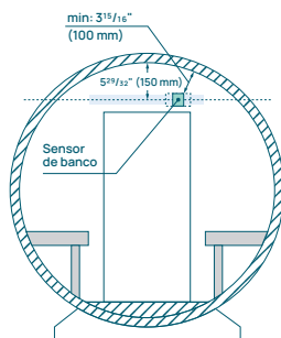
Figura 13. Instalación del sensor del banco en la sauna de barril, en la pared circular del extremo, en el lado opuesto al calentador.
