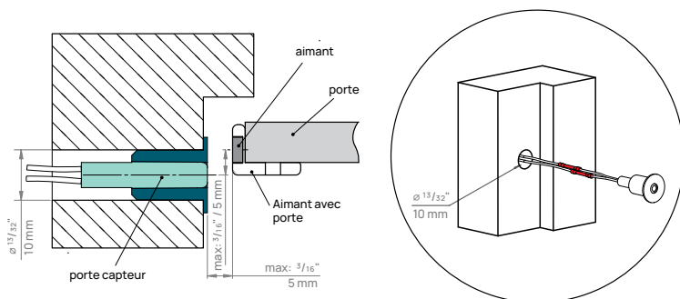
Figure 2. Emplacement du capteur de porte.
