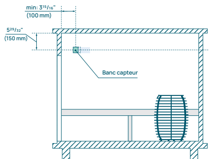
Figure 12. Installation du capteur de banc dans le sauna de type baril sur le mur incurvé, du côté opposé au chauffage.
