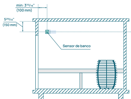
Figura 12. Instalación del sensor del banco en la sauna de barril en la pared curva, en el lado opuesto al calentador.
