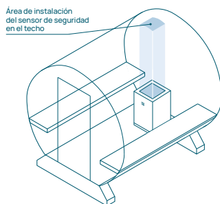
Figura 11. Instalación del sensor de seguridad en el techo de las saunas de barril: calentador montado en el piso.
