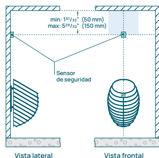
Figura 5. Instalación del sensor de seguridad en la pared: calentador montado en la pared
