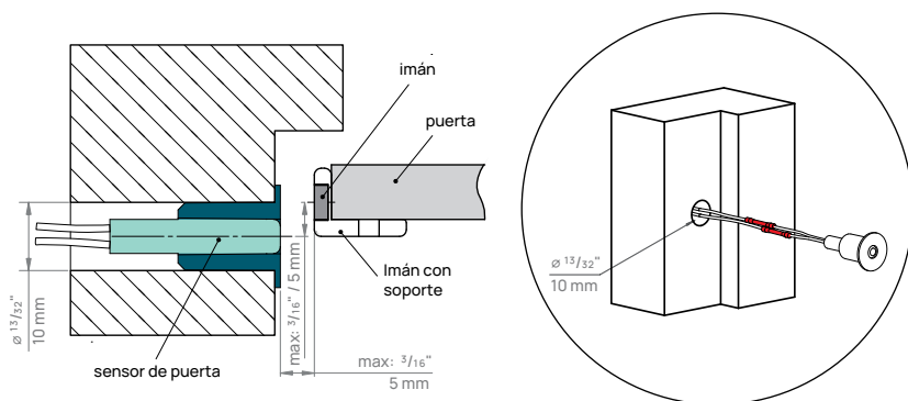
Figura 2. Colocación del sensor de la puerta.
