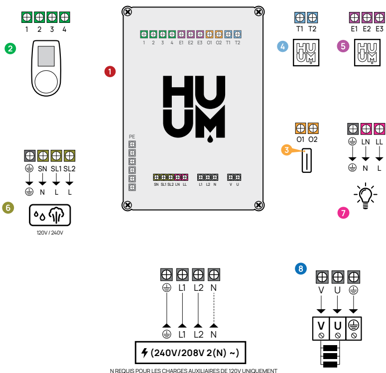
Figure 1. Raccordements électriques du chauffage.
