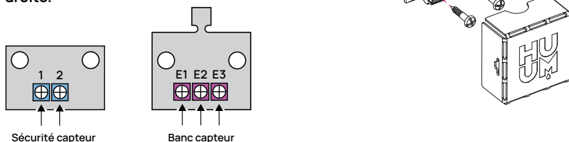
Figure 3. Installation du capteurs de sécurité et banc
