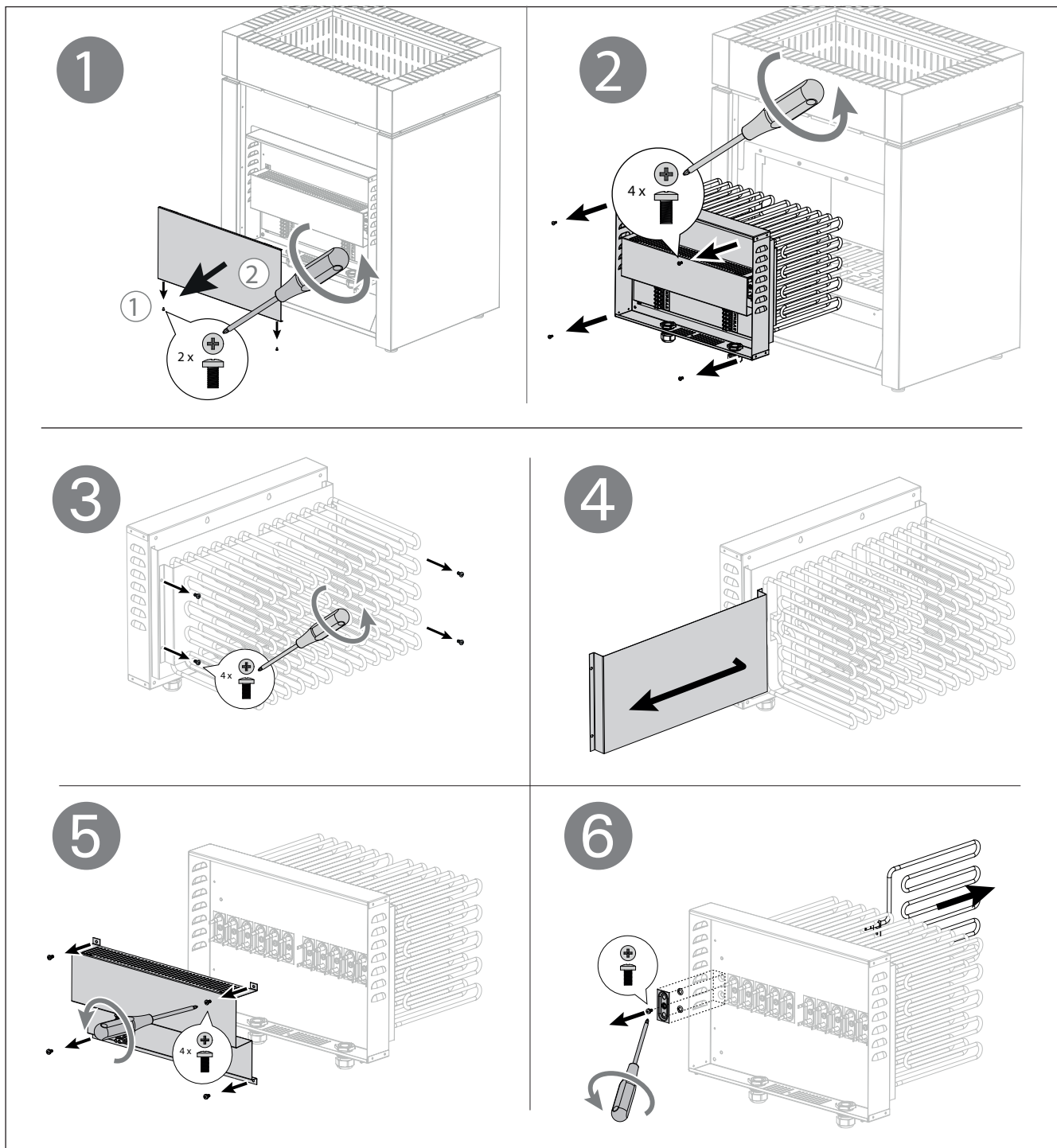
Kuva 6. Vastusten vaihtaminen Bild 6. Byte av värmelement
