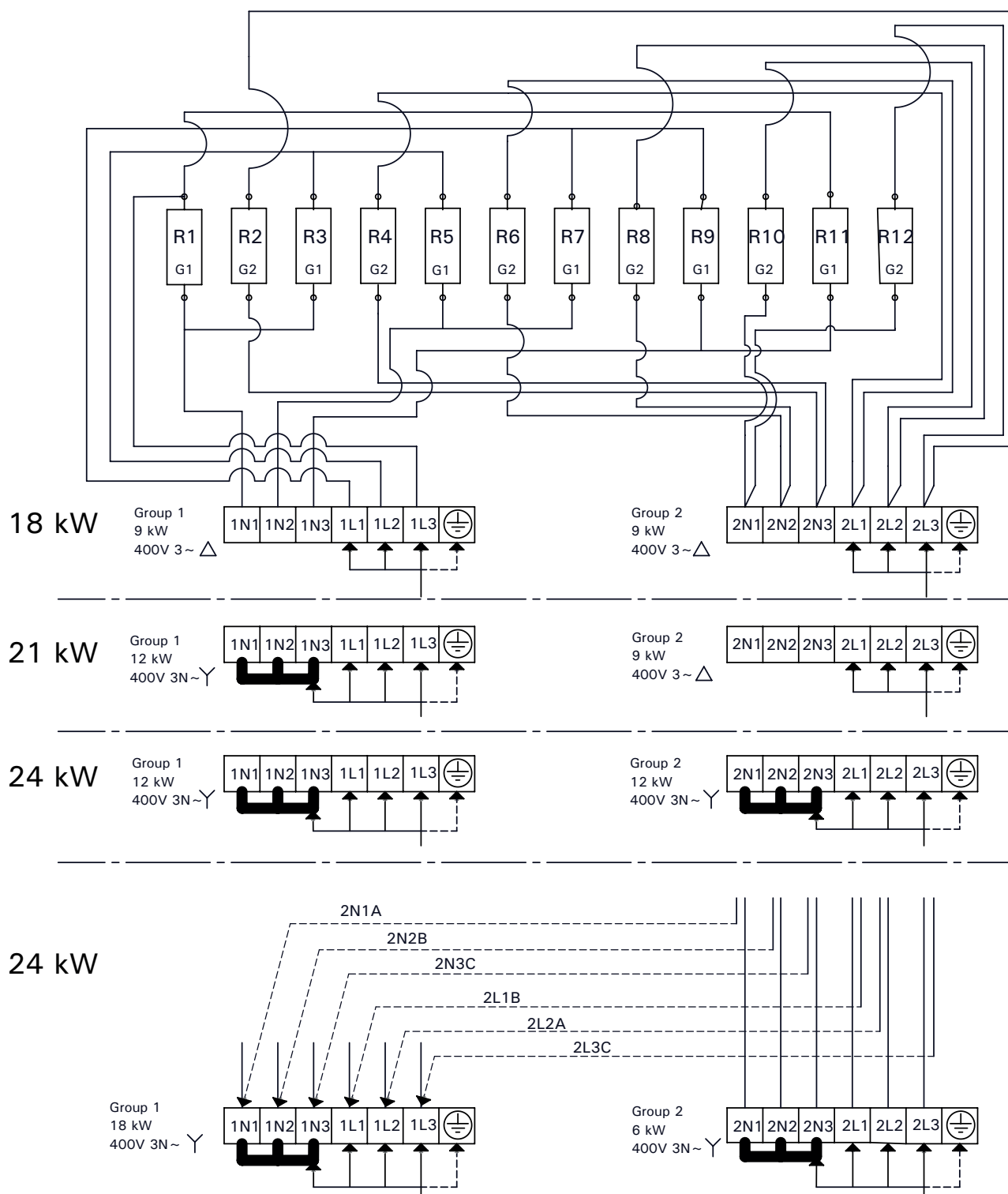
Рисунок 8. Электромонтаж каменки Joonis 8. Kerise elektriühenduse
