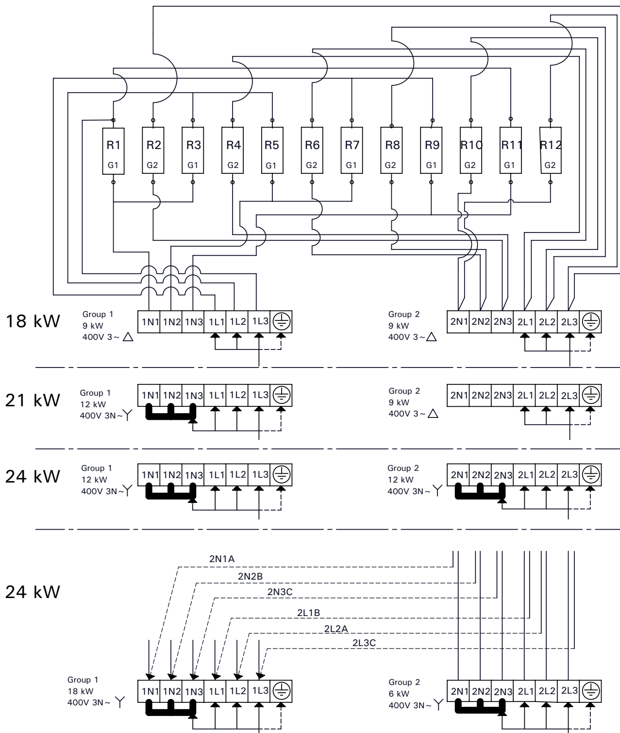
Figure 8. Connexions électriques
