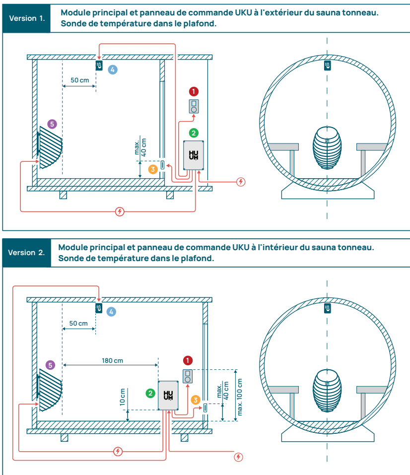
Figure 4. Installation de l'HUUM UKU dans les saunas tonneaux.
