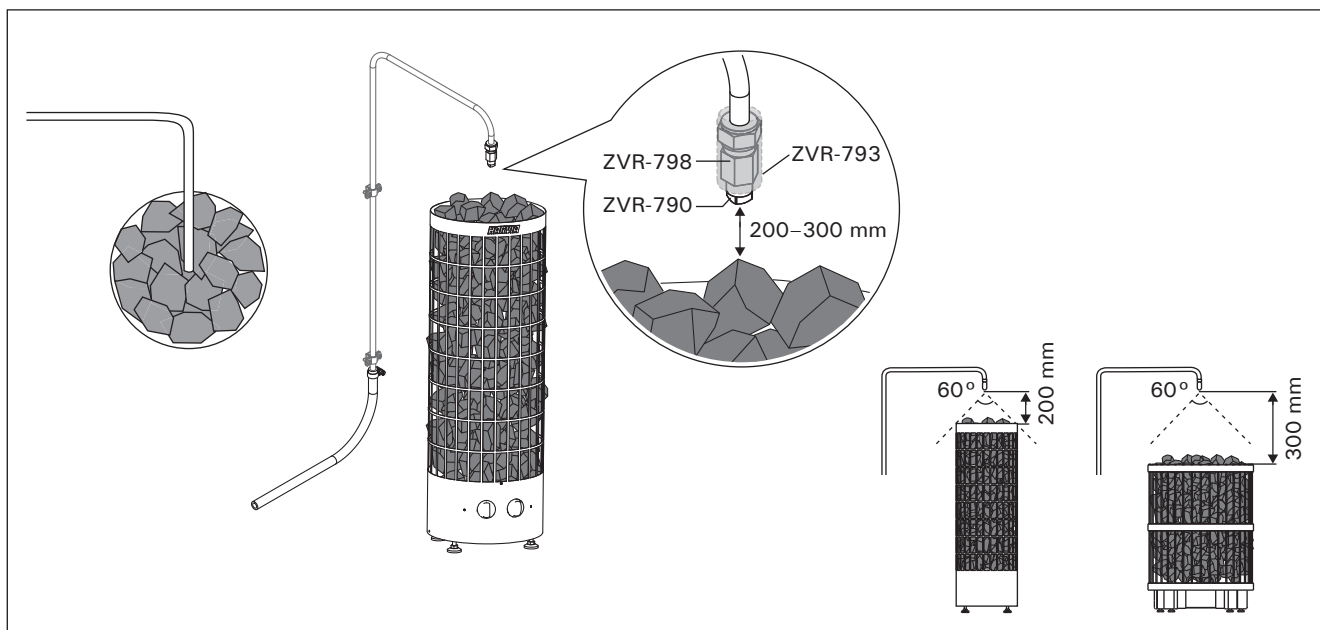
Kuva 4. Suuttimen asentaminen Bild 4. Montering av munstycke
