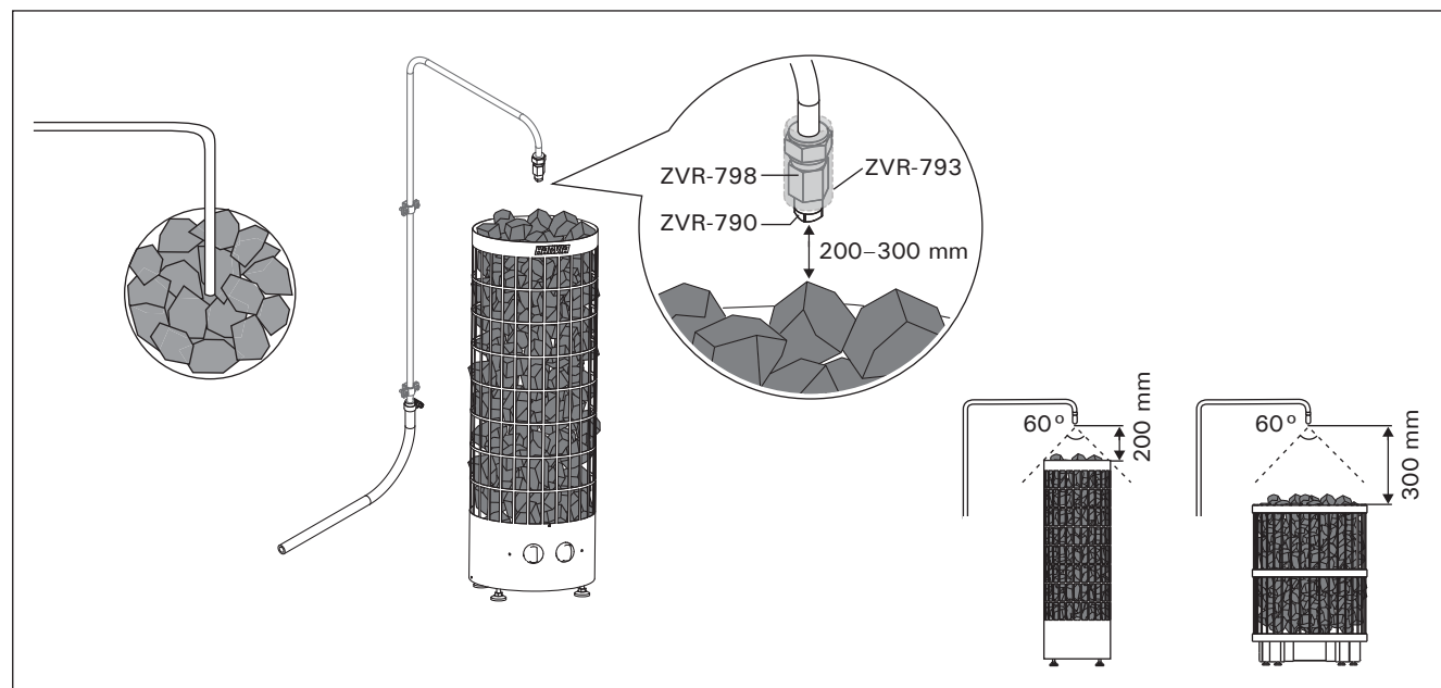
Рисунок 4. Установка сопла Joonis 4. Düüsi paigaldamine
