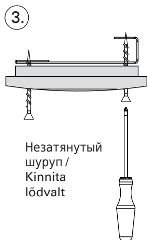
Рисунок 3б. Установка кнопок управления Joonis 3b. Juhtnuppude paigaldamine
