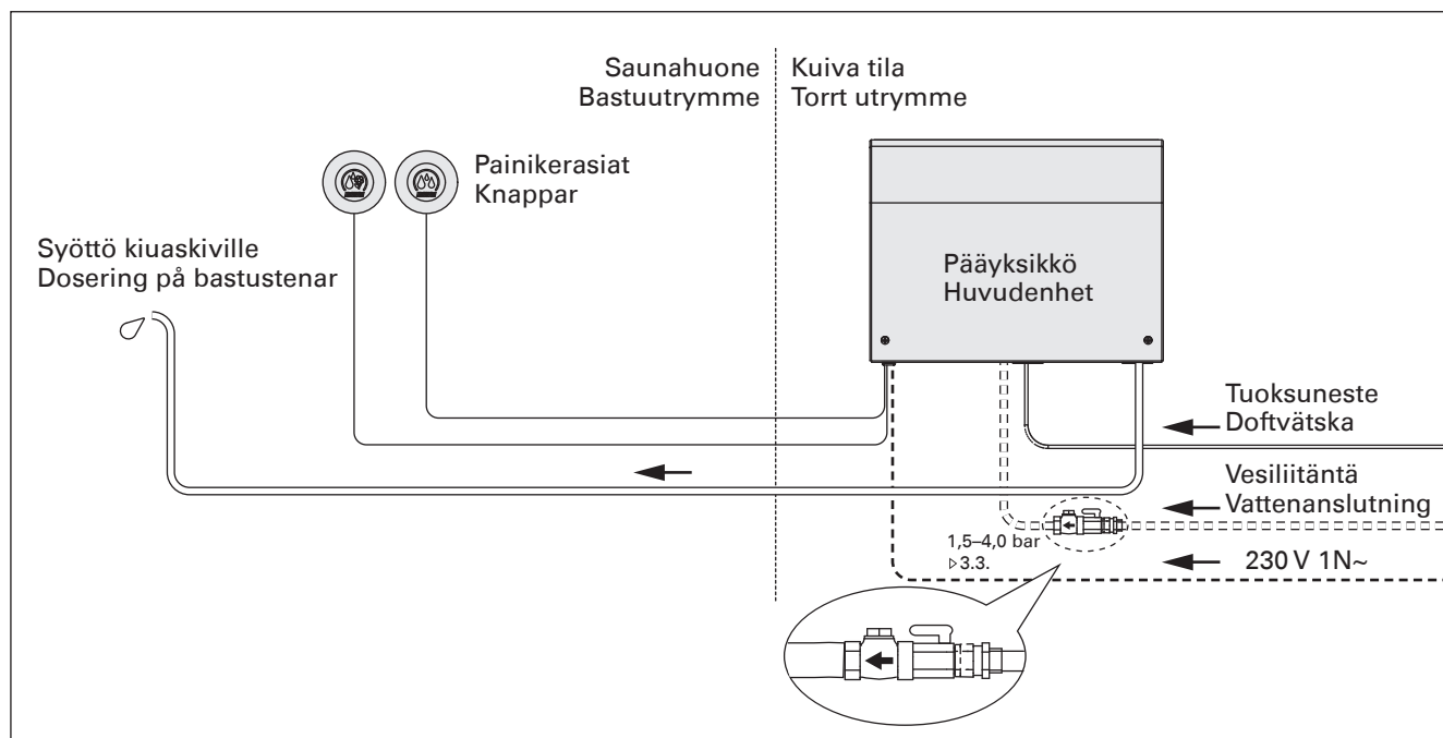
Kuva 1. Järjestelmän osat
