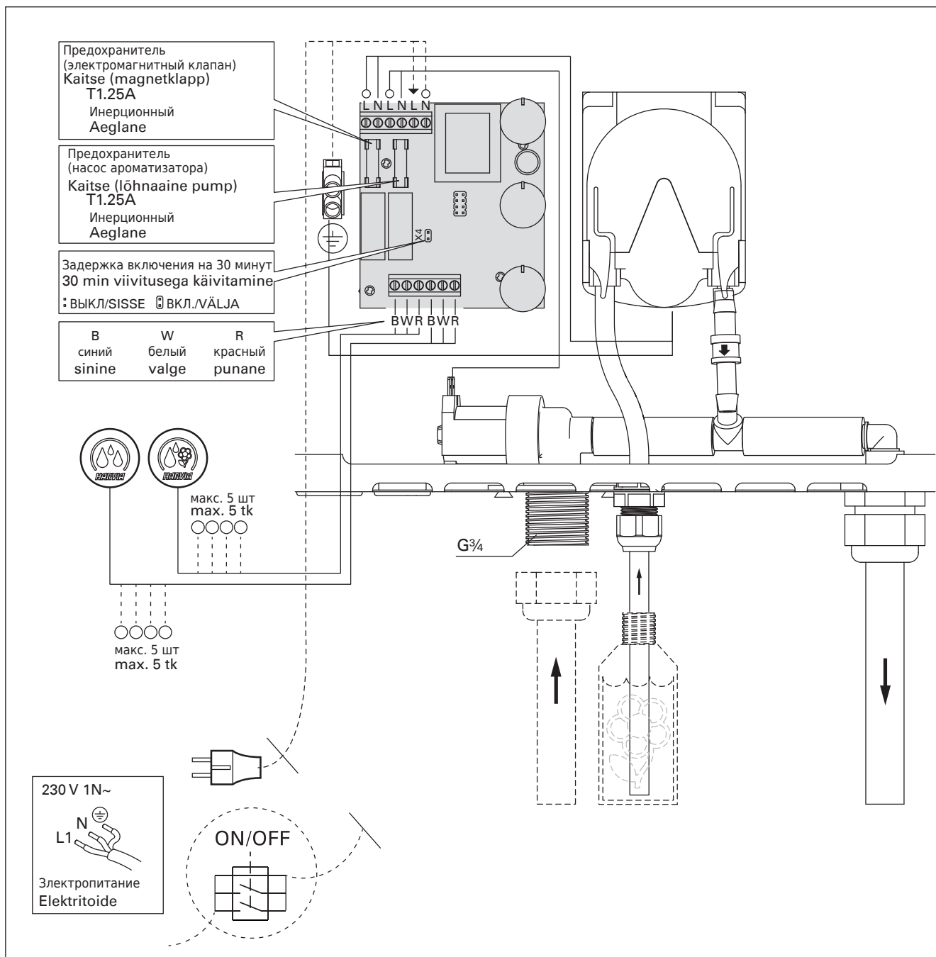
Рисунок 5. Соединения Joonis 5. Ühendused
